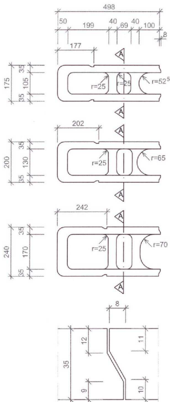
Draufsicht
