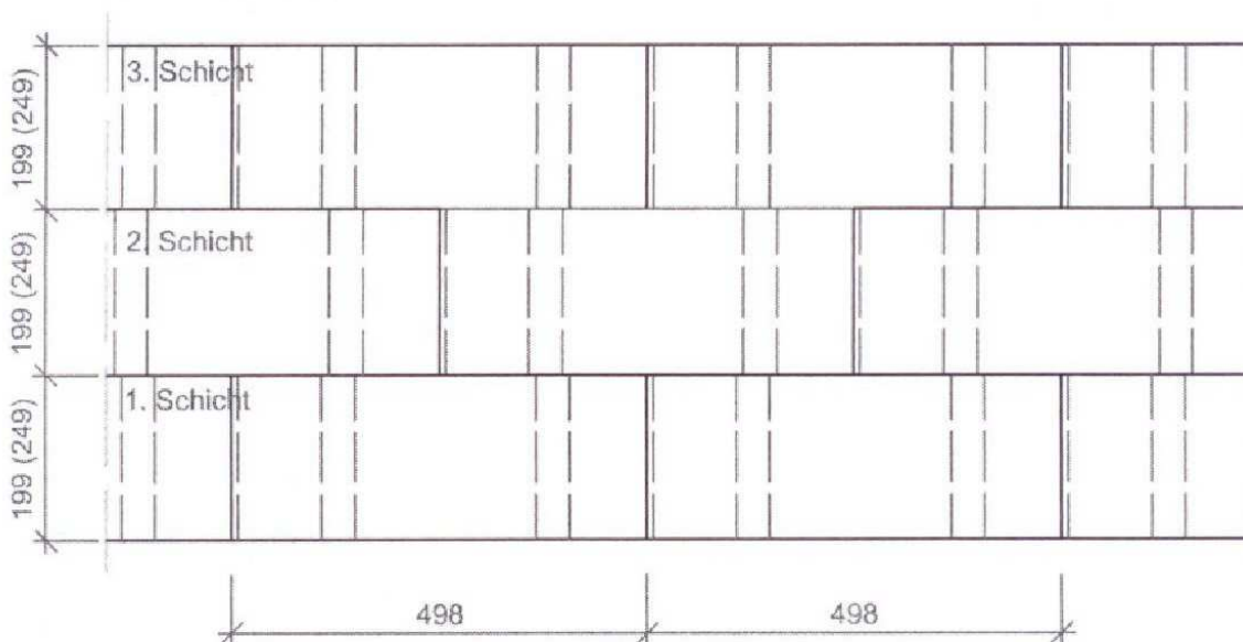
Wandansicht
