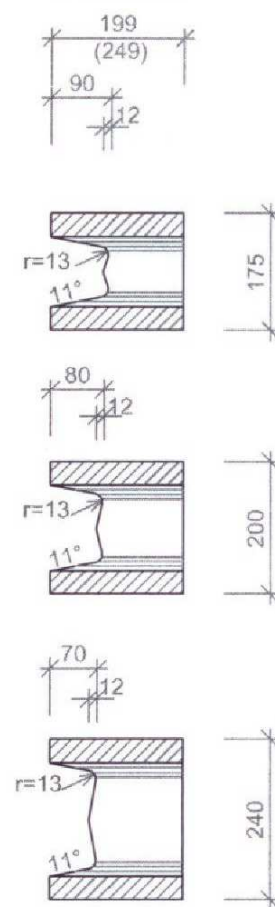
Schnitt A-A
