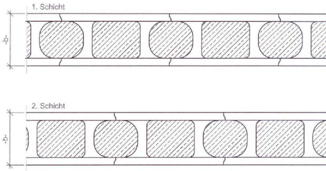
Draufsicht
