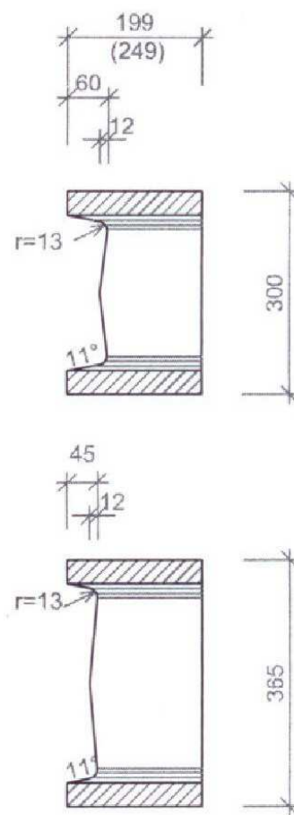
Schnitt A-A
