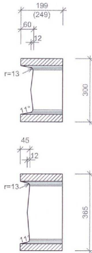
Schnitt A-A
