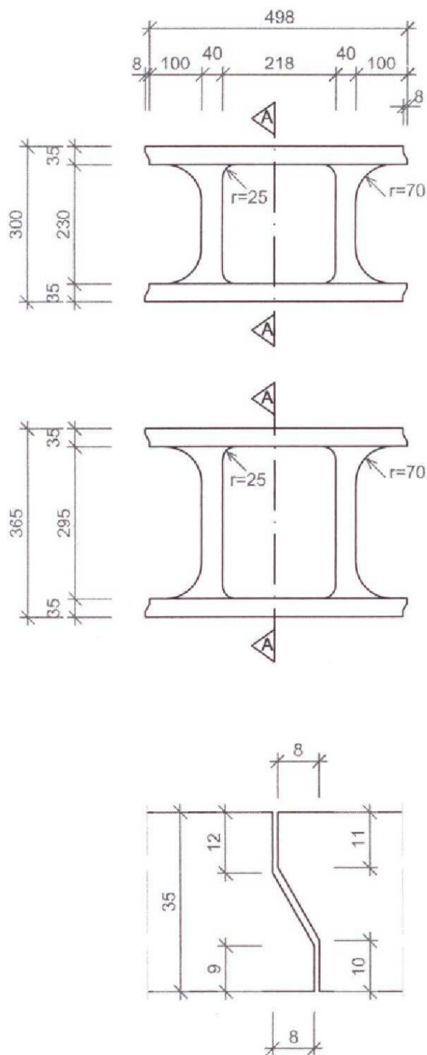
Draufsicht
