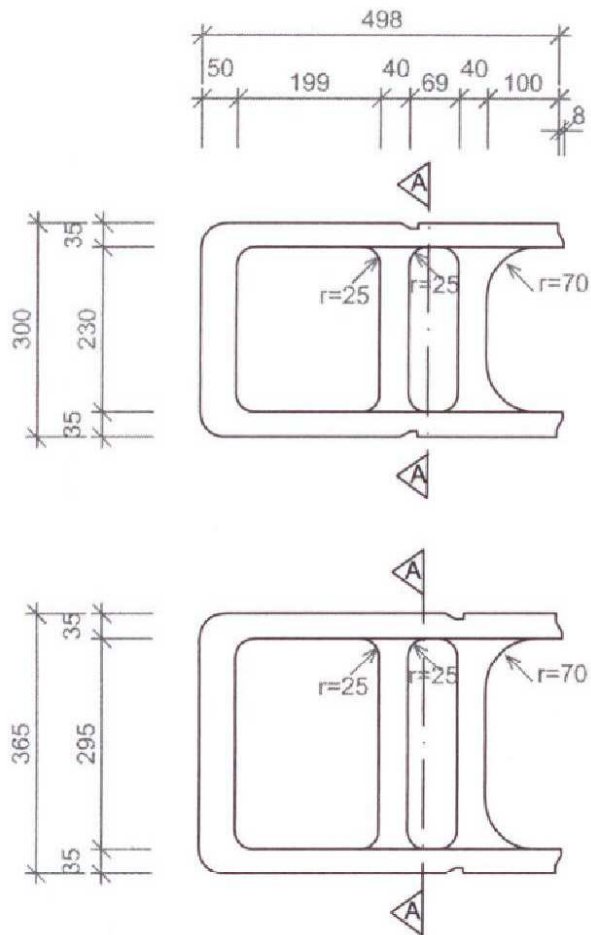
Draufsicht
